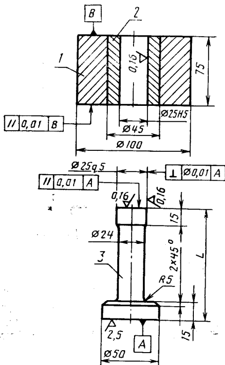
Пресс-форма для получения цилиндрических образцов диаметром 25 мм
